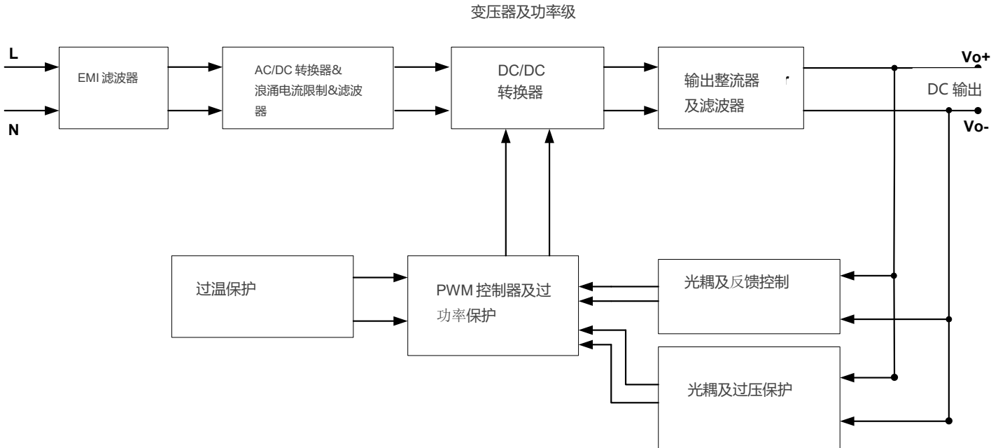
方块图
