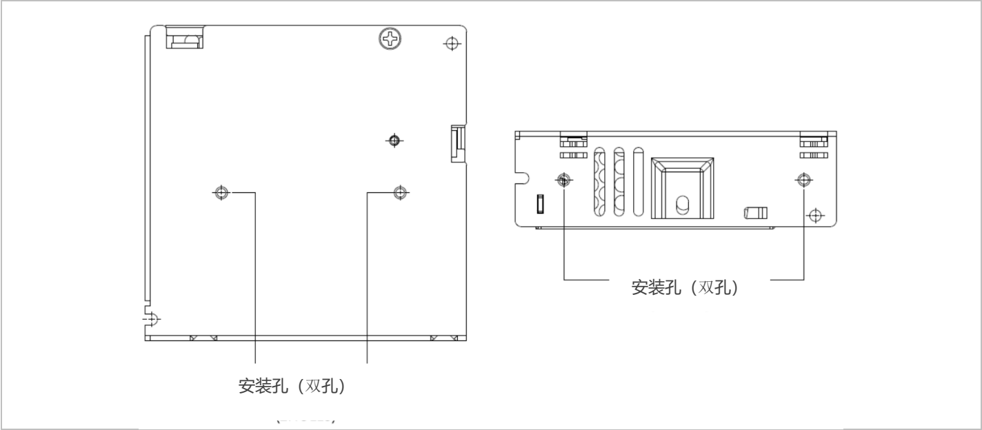
图 3 装配示意
