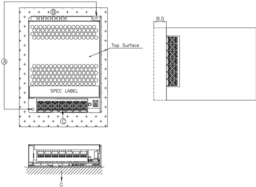
底面安装 (水平)
