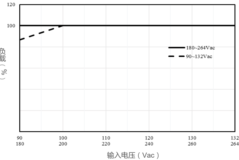
图 2 AC 输入电压降额 < 100 Vac 功率降额 1.33% / V
