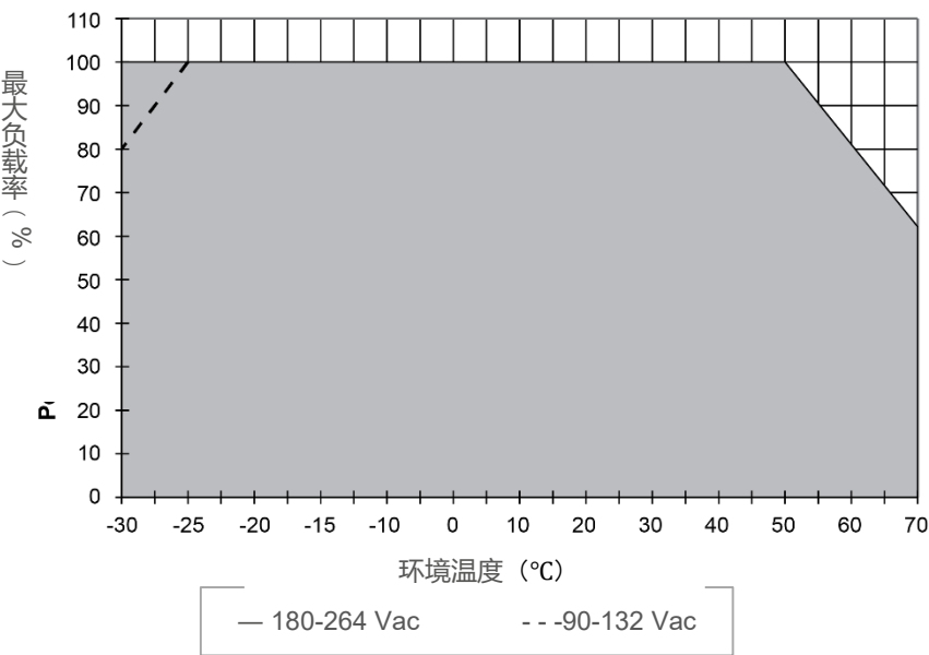
图 1 水平安装降额 < -25°C 功率降额 4.0% / °C @ 90-132 Vac > 50°C 功率降额 2.0% / °C
