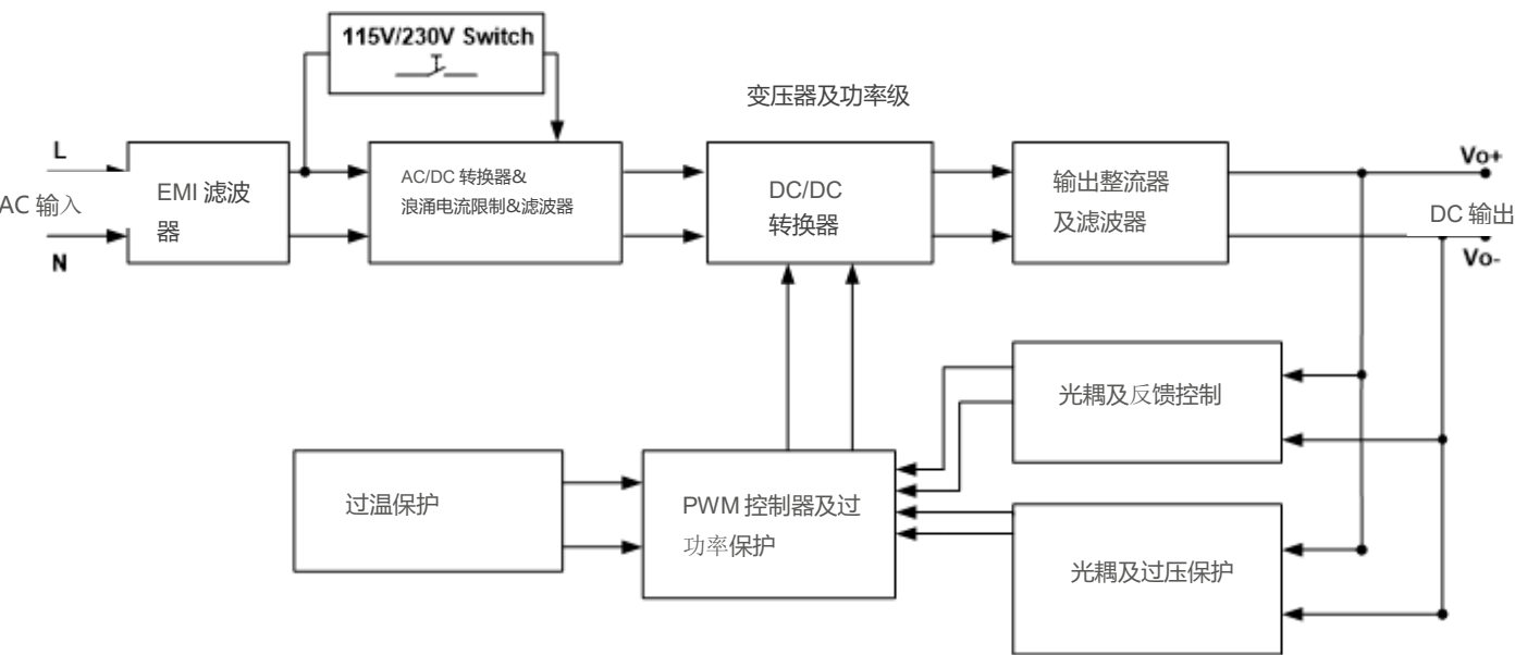
方块图
