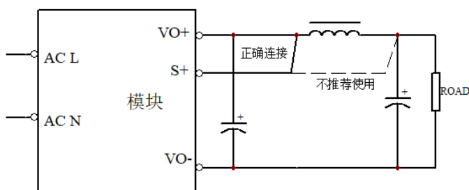
图 8 不推荐的连接方式
