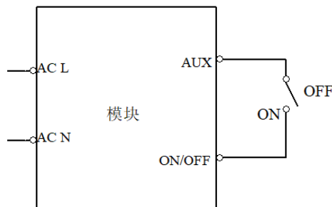
图 4 遥控接线图
