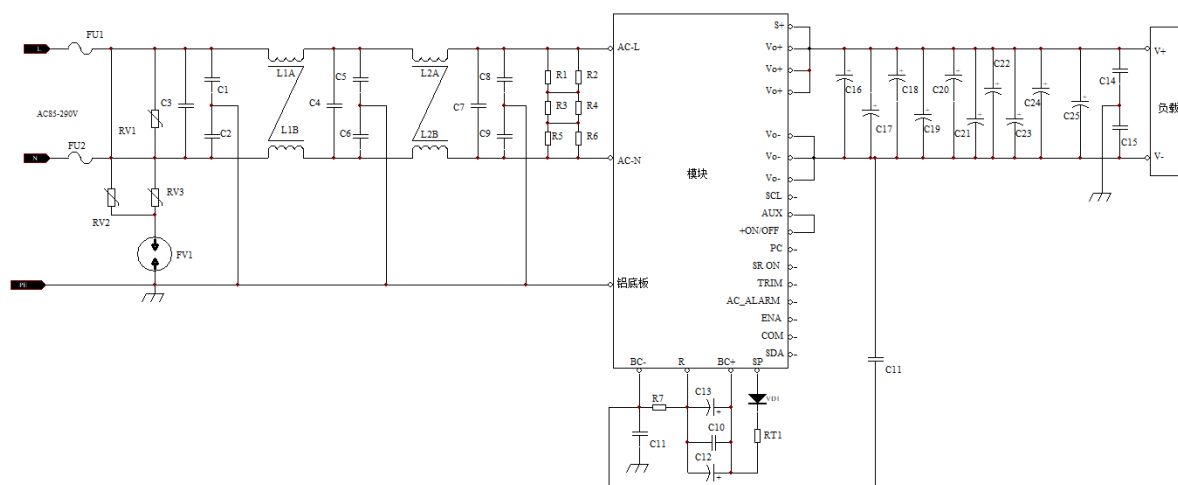
图 10 单机模块外围电路接线图
