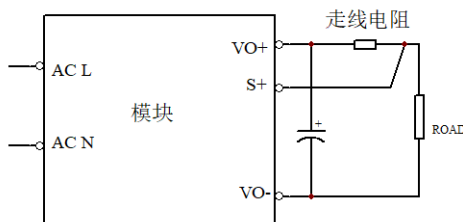
图 6 远端补偿电路
