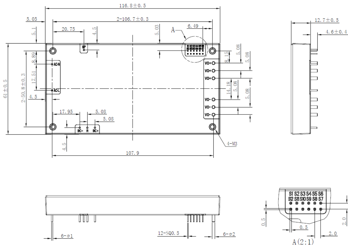
图 3 模块结构图
