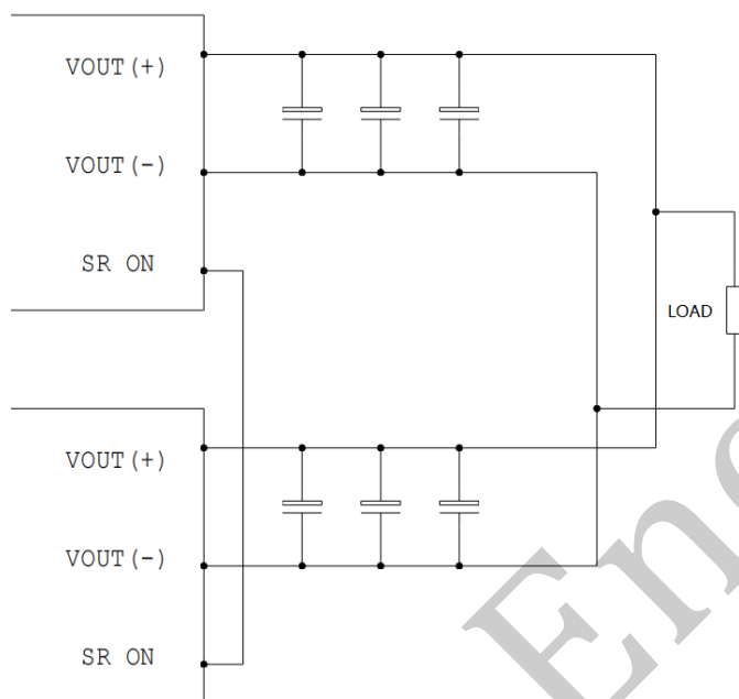
并联同步起机连接图
