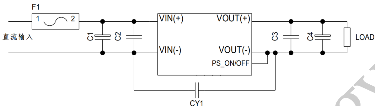
单机模块外围电路接线图
