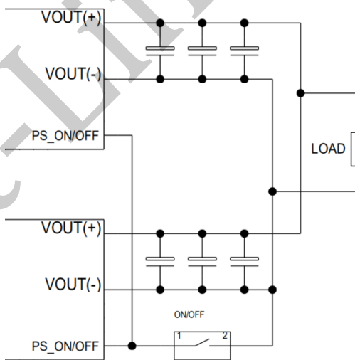
并联使用连接图
