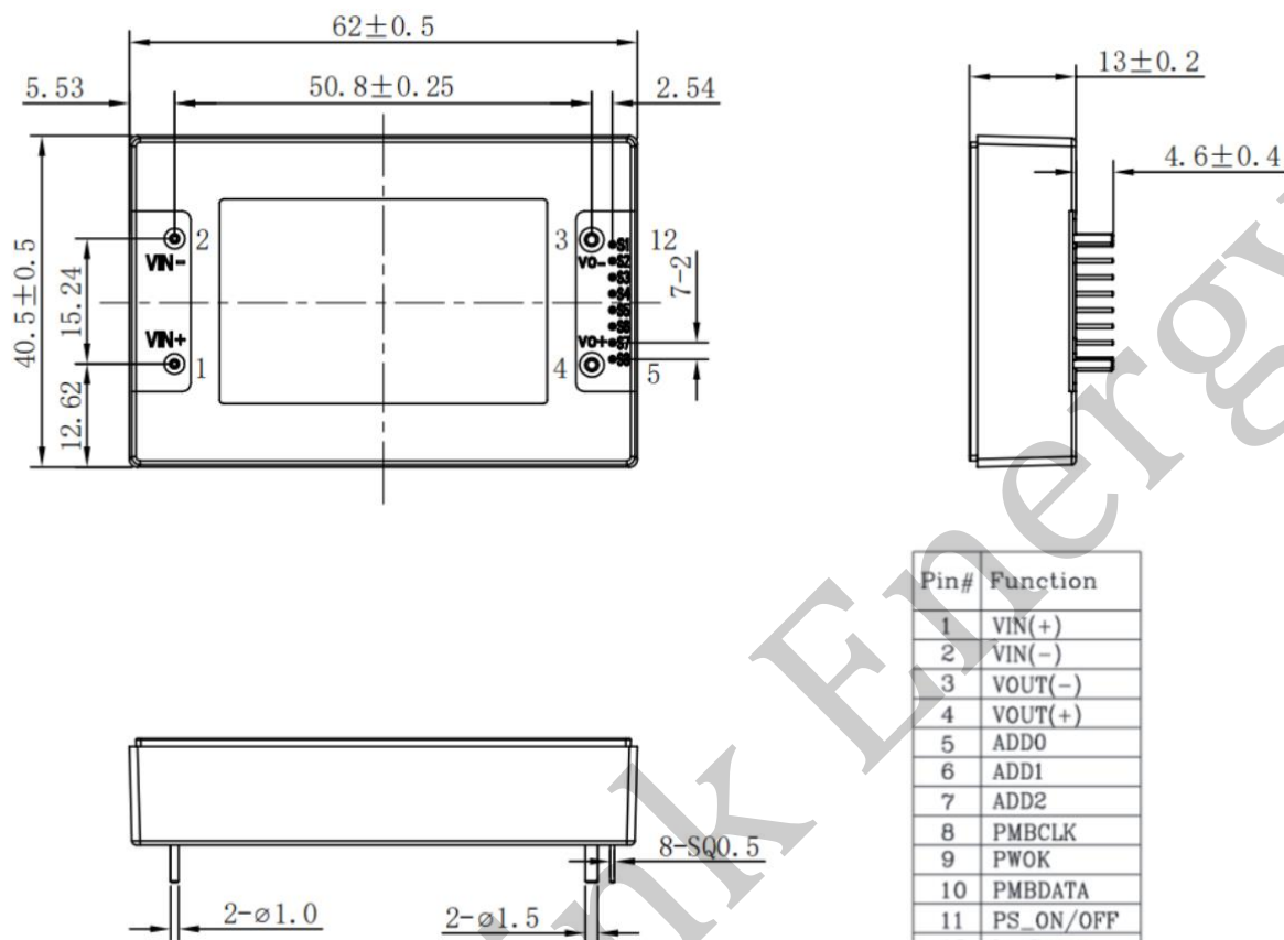
模块结构图
