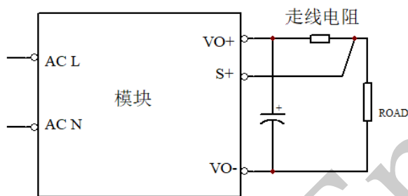
图 6 远端补偿电路
