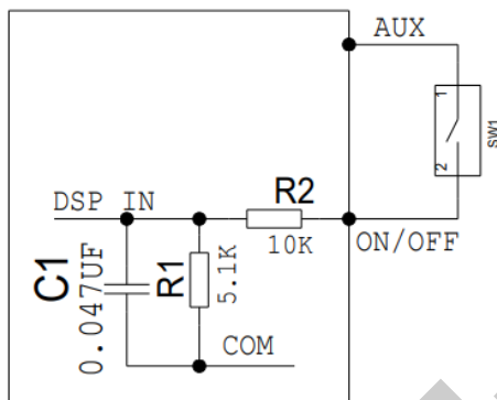
图 4 遥控接线图
