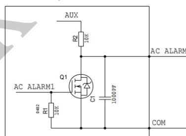
图 12 AC ALARM 端子模块内部电路
