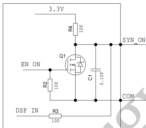
图 10 同步端子 SYN ON 模块内部接线图
