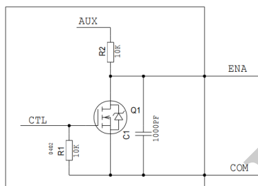
图 11 ENA 端子模块内部电路
