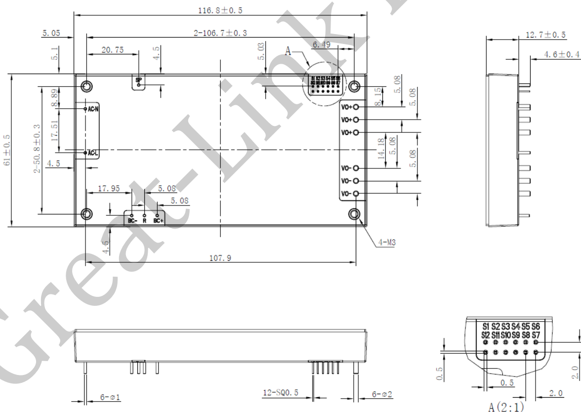
图 3 模块结构图
