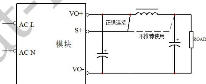
图 8 不推荐的连接方式
