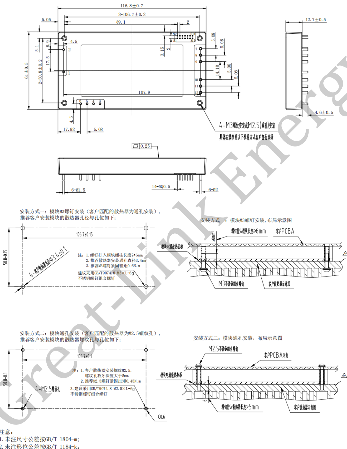
图 3 模块结构图
