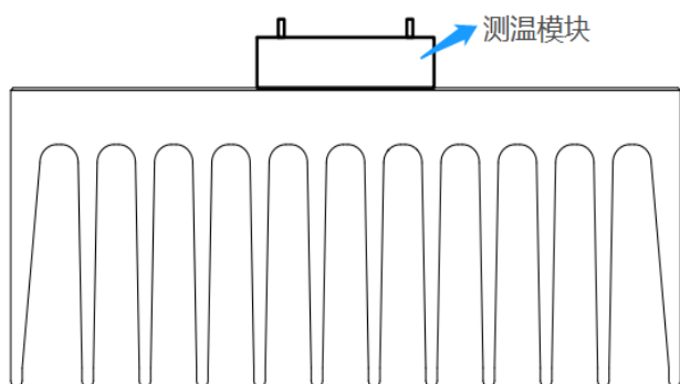
图 13 模块铝基板热点温度位置示意图
