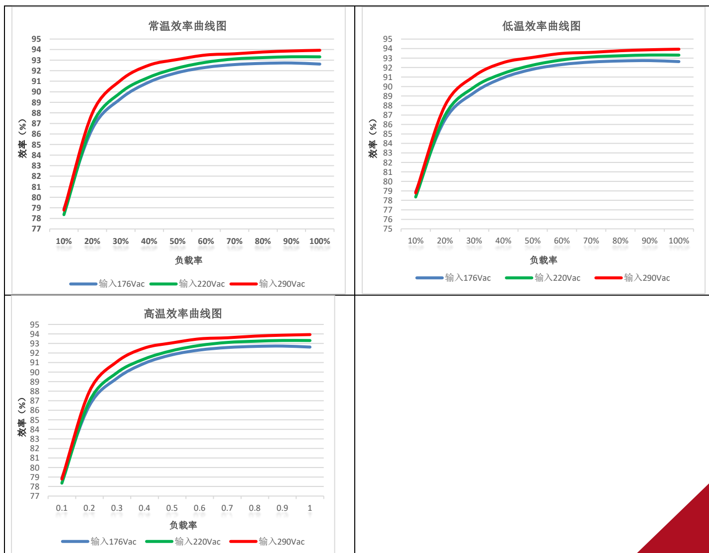
图 2 效率特性曲线图
