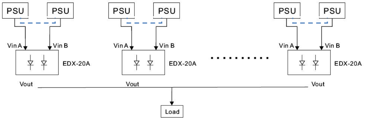
3.4 可靠性系统构建图 Reliability system:
